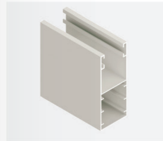
PVC VODILICA (53x22)
